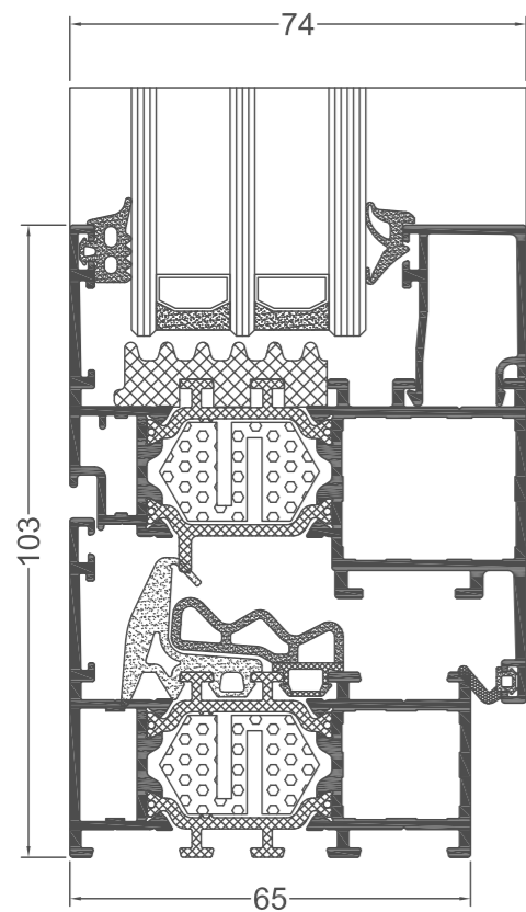
izolația termică depinde de combinația de profile și grosimea umpluturii Fereastra Genesis 65 (GR010 + GR020)
