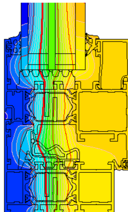
exemplu de distribuție izoterma pentru combinația toc cercevea de fereastră din sistemul GR 65 (GR010 + GR020)
