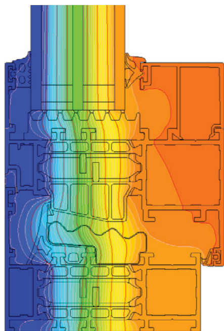
exemplu de distribuție izotermă pentru combinația toc cercevea fereastră cu sistemul GN 75 (GN010 + GN020)
